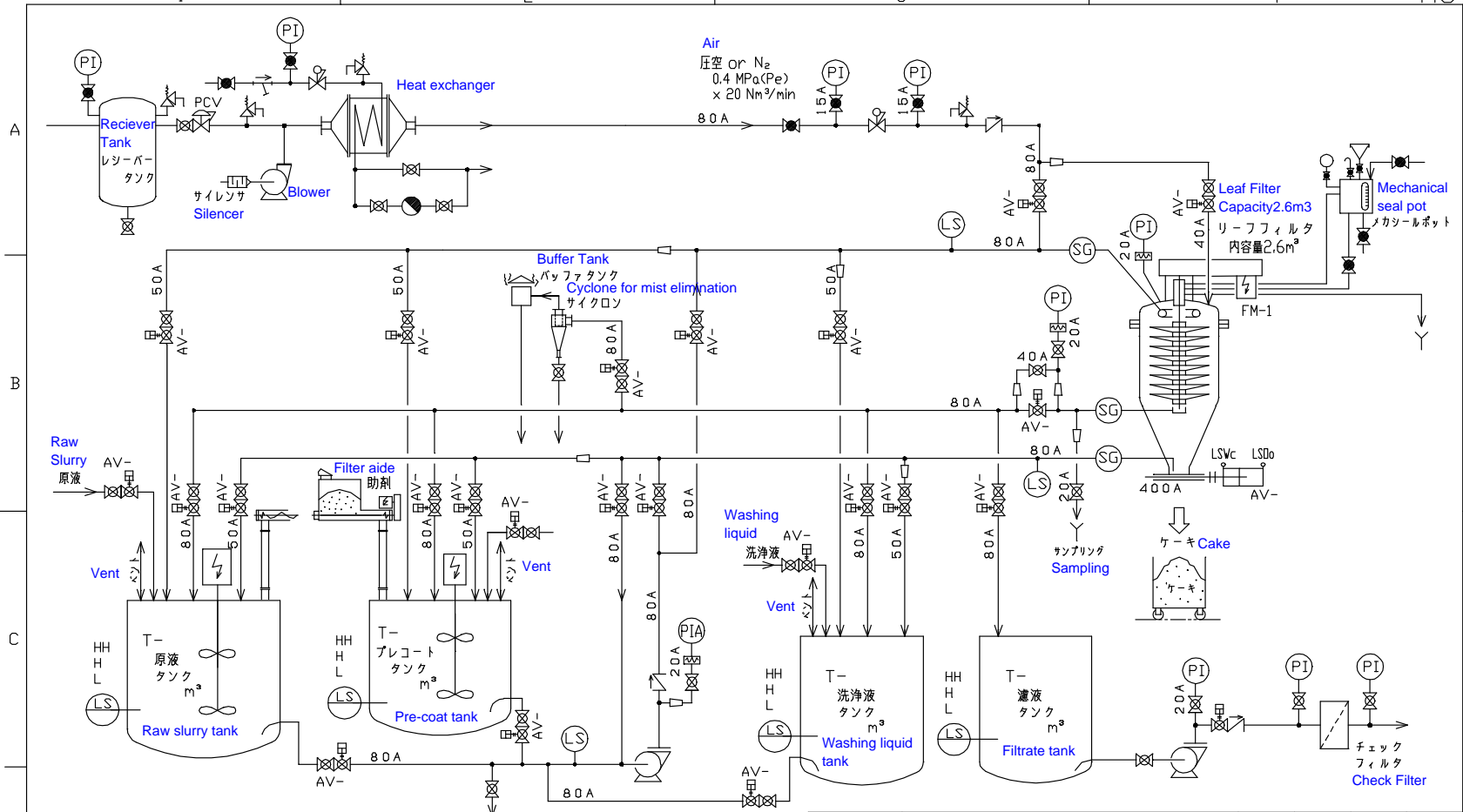
P-1 フィルタポンプ Filter Pump 25m³/Hr x 40m
